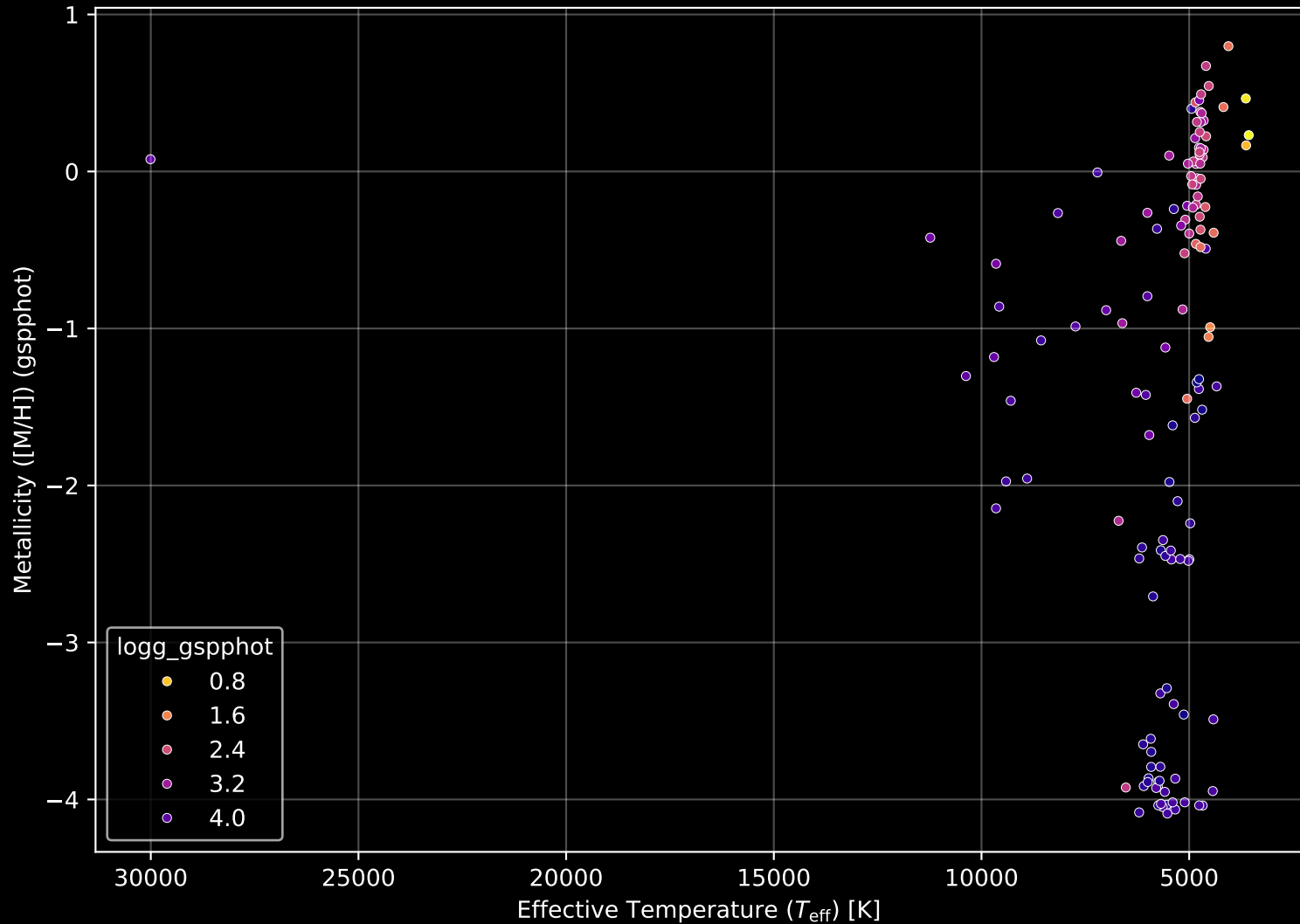
APOGEE DR17 Field: [005+03-O] Stellar Population Parameters (n= 136)
